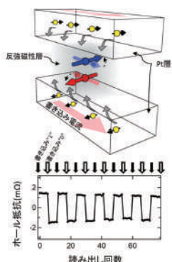
反強磁性体磁気メモリの実証
