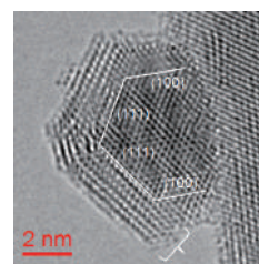
排気ガス浄化触媒金属粒子の原子レベル反応その場観察
