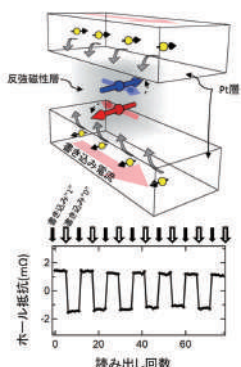
反強磁性体磁気メモリの実証
