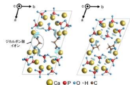
リン酸ハカルシウム: \text{H}_2\text{O} の有無が原子・電子構造に与える影響
